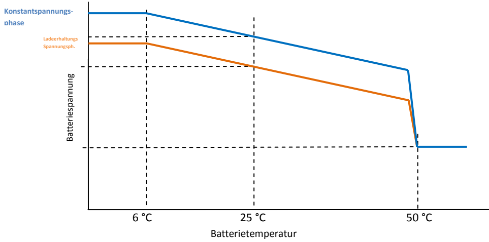
Abbildung 1: Temperaturkompensationskurve
